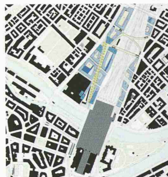
Das städtebauliche Konzept HB Zürich: Verlängerung der Strassen bis an die Gleise, ein Boulevard mit zwei Plätzen und eine Fussgängerpasserelle (Plan: Amt für Städtebau, Zürich)
