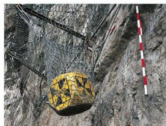
Test bestanden – der Prüfkörper hängt im Netz (Bild: Autor). Rechts: Bremsringe ziehen sich bei grosser Kräfteinwirkung zusammen (Bild: Geobrugg)
