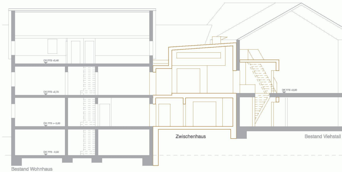
07 Schnitt durch das Ensemble: Verzahnung des Neubaus mit den Außenmauern des Bestands. Die neue Treppe im Viehstall ermöglicht eine räumliche Abkoppelung der Wohnung im Obergeschoss des Neubaus (Mst. 1:200)
