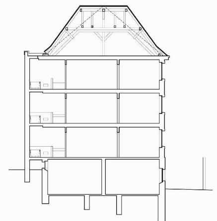
Areal 1, 1. Rang: Querschnitt mit Erweiterung
