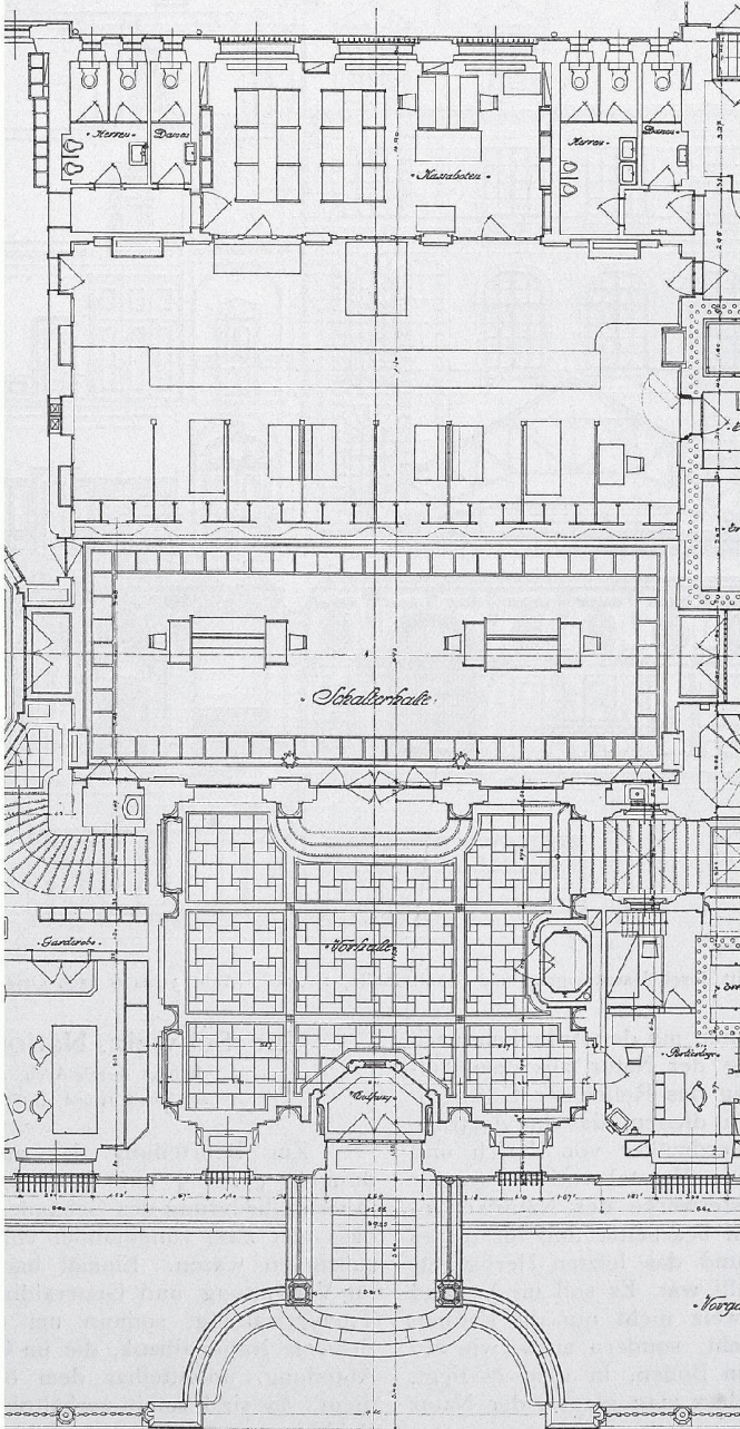
Die Schweiz. Nationalbank in Bern. — Grundriss vom Erdgeschoss. — Mass
