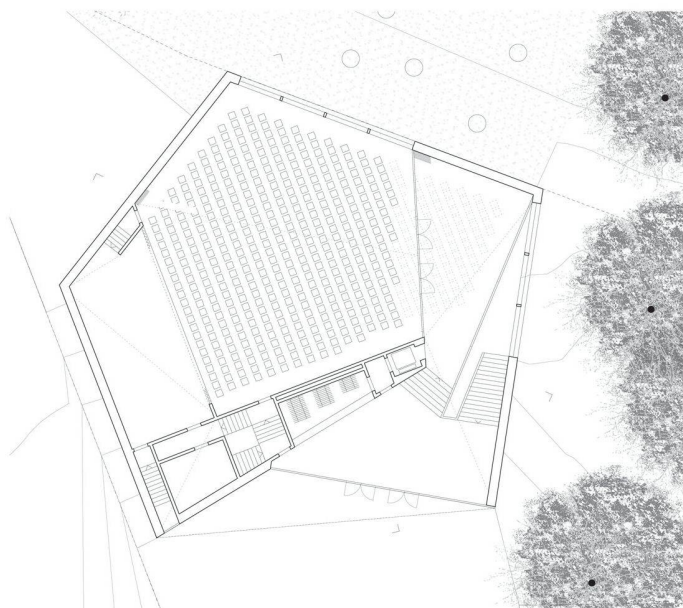
03 Grundriss Eingangsgeschoss mit Saal für 500 Personen, Mst. 1:500
