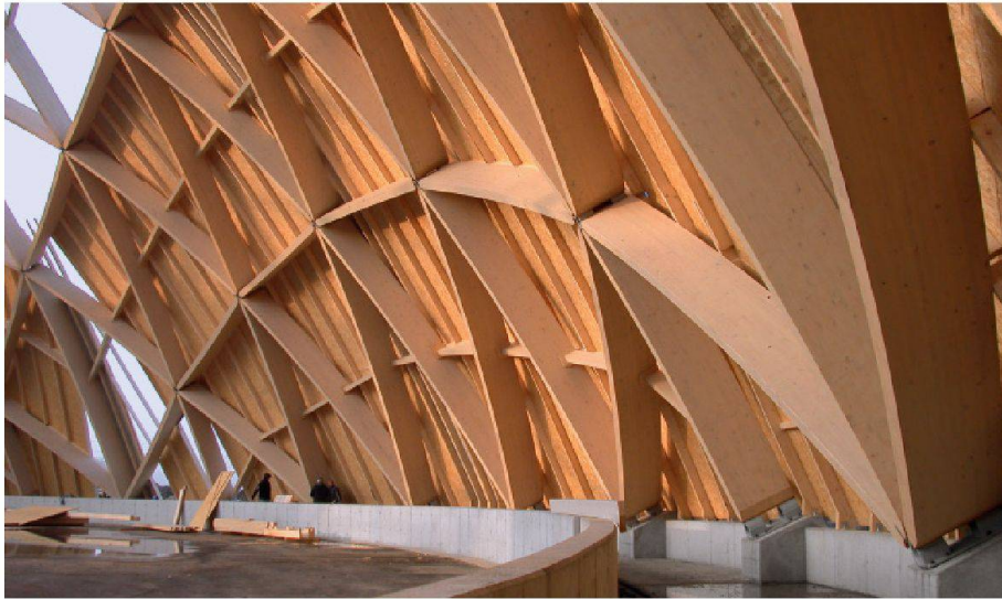
01 Innovativer Ingenieurholzbau: Saldome, Möhlin (Häring & Co AG, Pratteln) (Foto: Jürg Fischer)
