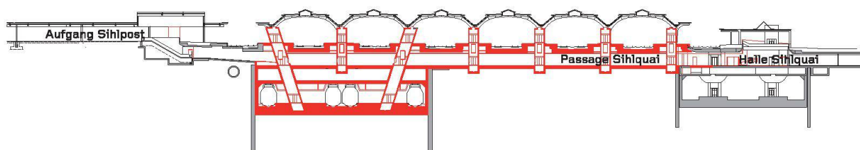
11 Querschnitt Passage Sihlquai, Mst. 1:1500
