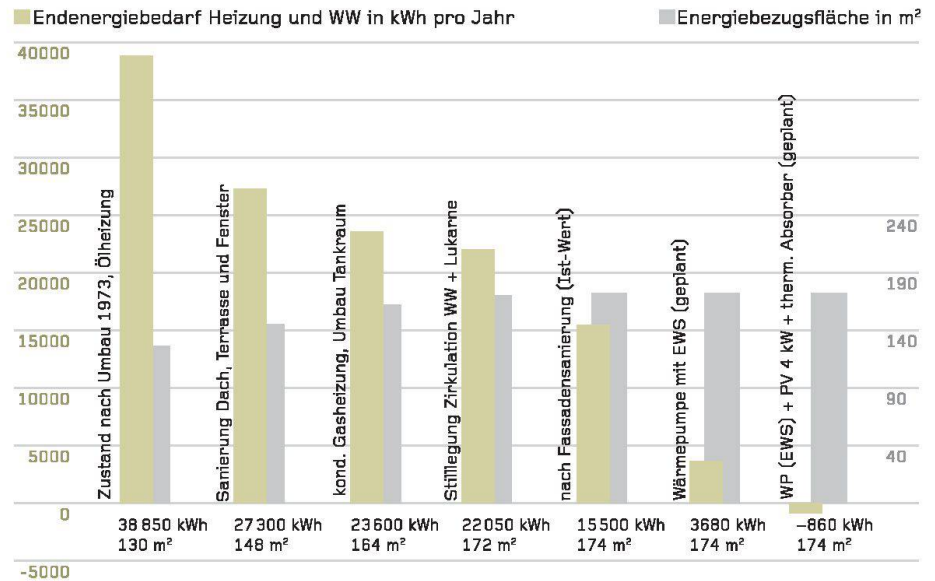
03 Entwicklung von Endenergiebedarf für Heizung und Warmwasser sowie Energiebezugsfläche nach den einzelnen Schritten der etappenweisen Sanierung. (Grafiken: Autor)
