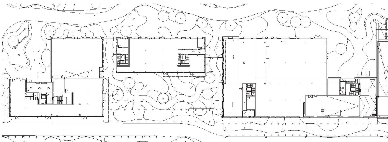
02 Erdgeschoss
