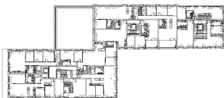
2. Obergeschoss
