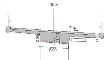
3. Preis: «Vulp»: 8-feldriger Spannbeton-Balkenträger ( l/h = 28 ) mit rechteckigen Pfeilern von identischem Querschnitt.
