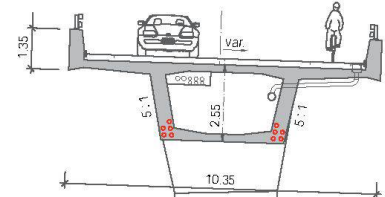
2. Preis: «Rabius»: 3-feldriger, gevouteter Spannbeton-Hohlkastenträger ( l/h = 18-32 ) mit zweifach konischen Pfeilern.
