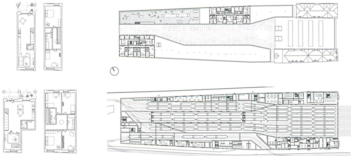
Maisonetten über dem Depot. Mst. 1:500.
