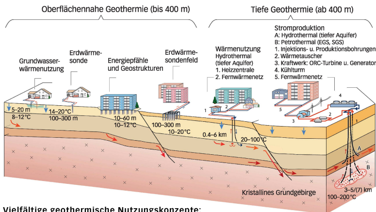
Vielfältige geothermische Nutzungskonzepte: Oberflächennahe, untefe Geothermie nutzt Erdwärme bis etwa 400 m.
