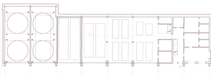
«Yuki»: Grundriss Erdgeschoss, Mst.1:600.
