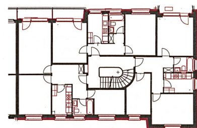
Grundriss, Massstab 1:400.
