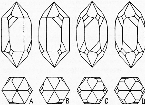
Fig. 23. Charakteristische Symmetrie des Quarzes, Links- (A, C) und Rechtsquarz (B, D). Zwillinge (C, D).
