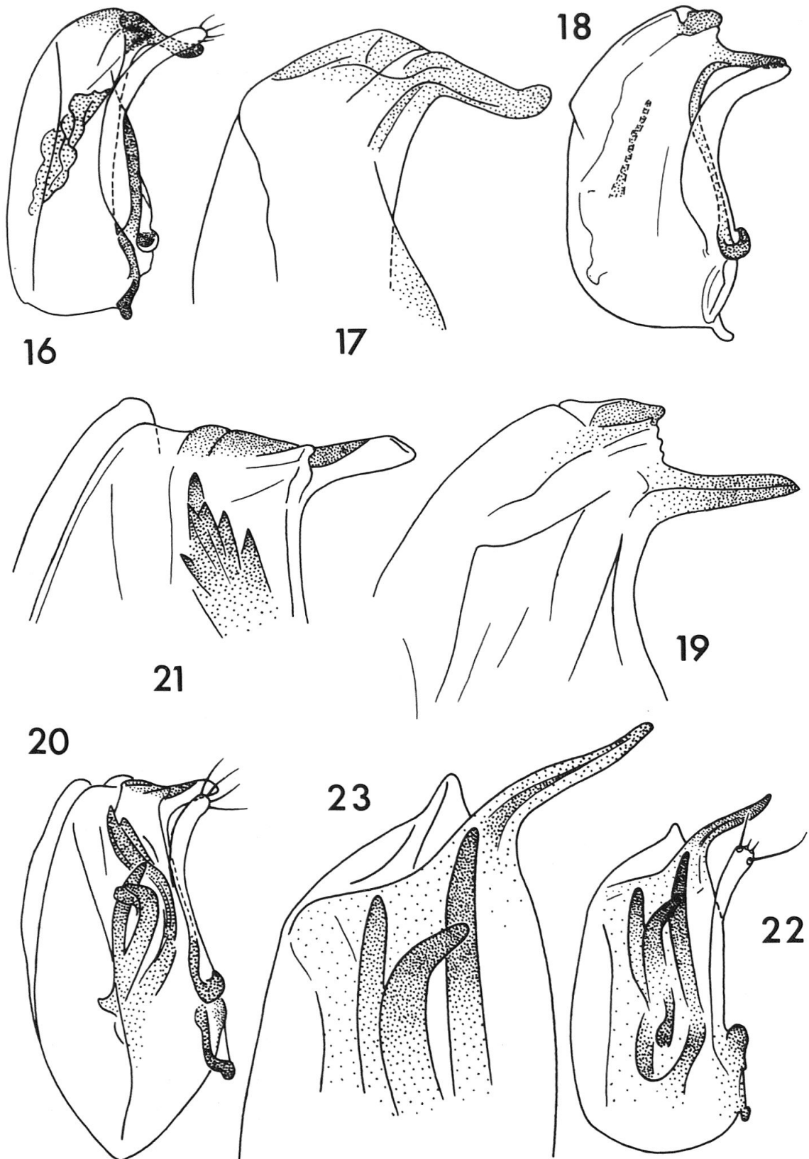
Fig. 16-23: Listriophorus typicus n. sp., édéage de profil (16) et détail du profil de l'éédéage (17); L. rarus n. sp., édéage de profil (18) et détail du profil de l'éédéage (19); L. beaumonti n. sp., édéage de profil (20) et détail du profil de l'éédéage (21); L. myops n. sp., édéage de profil (22) et détail du profil de l'éédéage (23).
