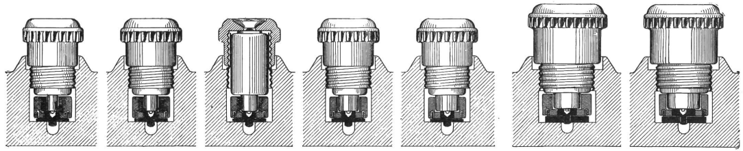
Normales Edisongewinde 6 grün 10 rot 15 grau 20 blau 25 gelb 35 schwarz 60 Ampère kupfer Grosses Edisongewinde Farbe der Kennvorrichtung Normal-Diazed der S. S. W. und Type P. D. von V. & H. A.-G.
