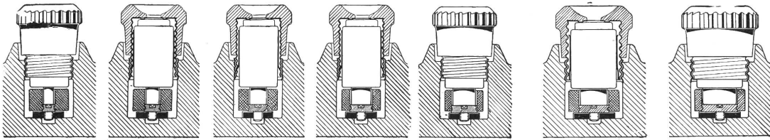
Normales Edisongewinde 6 grün 10 rot 15 grau 20 blau 25 gelb 35 schwarz 60 Ampère kupfer Grosses Edisongewinde Farbe der Kennvorrichtung Type D. der A. E. G.
