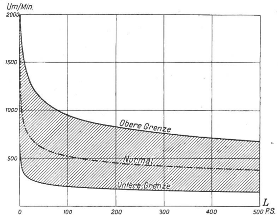
Abbildung 5. Rechnungsmässig ermittelte Kurven der Umdrehungszahl zur Vergleich der Kurven nach Abbildung 1 mit der Formel (5).
