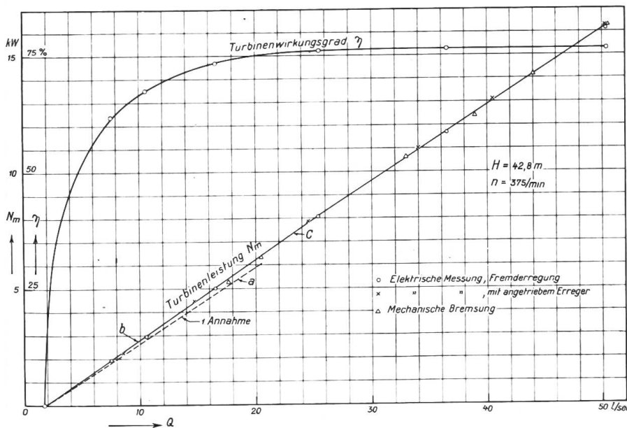
Fig. 1. Leistung und Wirkungsgrad der untersuchten Freistrahlturbine bei konstantem Gefälle.
