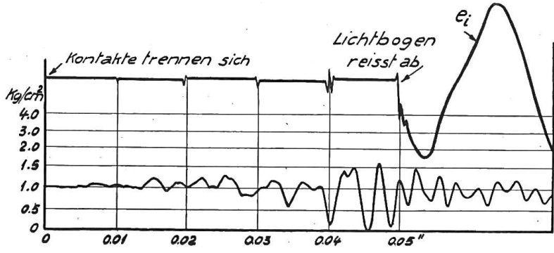
Fig. 4. Druckverlauf im Innern des Oelschalters. Statischer Druck = Atmosphärendruck.
