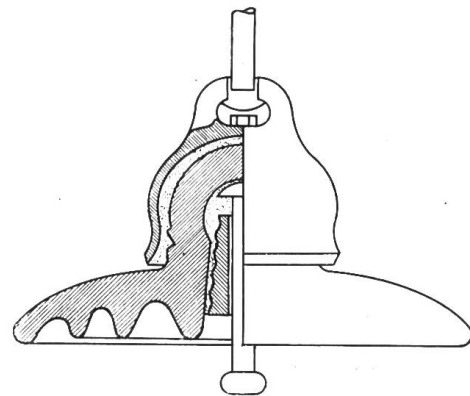
Fig. 4 Untra-Isolator.
