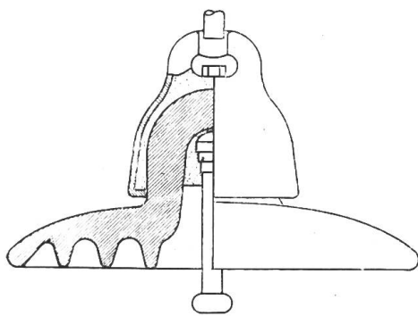
Fig. 3 Kapfen-Isolator.
