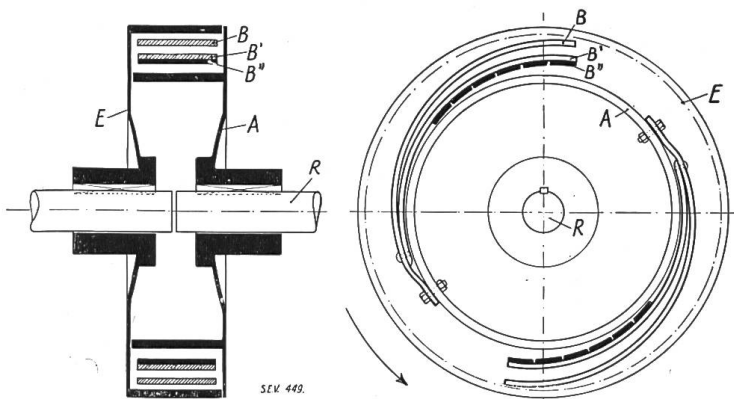
Fig. 10. Schematische Darstellung der Kupplung I. R: Rotorwelle A: Antreibender Teil } der Kupplung. E: Angetriebener Teil B und B': Lederriemen. B'': Blechstreifen.
