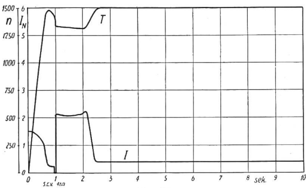
Fig. 27. Kupplung IV.
