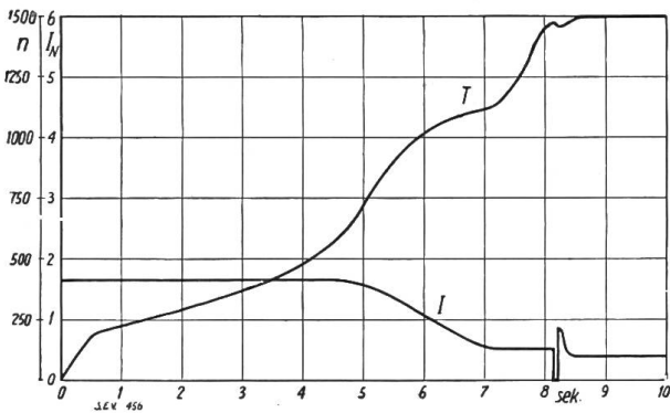
Fig. 19. Kupplung II.
