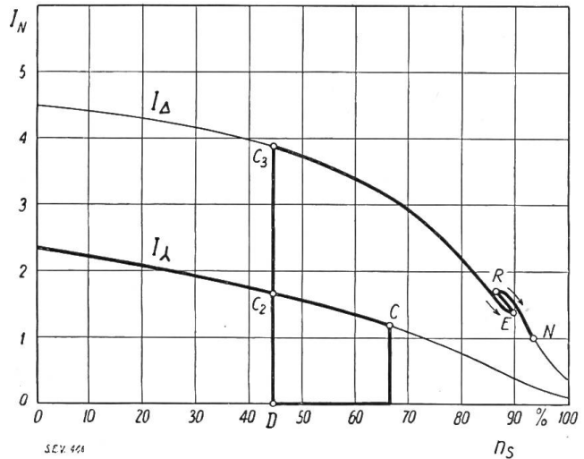
Fig. 7 a (oben) und 7 b (unten). Anlaufvorgang bei reinen Fliehkraft-Kupplungen in Funktion der Tourenzahl. Kurve M_K : Durch die Kupplung bei Gleiten übertragbares Moment. Kurve OR : Durch die Kupplung bei Haftreibung übertragbares Moment.
