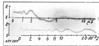
Fig. 6. Umgewandelte Welle u an einer zweilagigen, gegenläufigen Zylinderspule nach Fig. 5. e = 2600 V. U_0 = 5200 V. Stirnlänge S_0 \sim 3 m.
