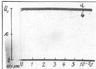
Fig. 4. Umwandlung einer Sprungwelle an einer vielspulgigen Zylinderwicklung (Scheibenwicklung, 4 Doppelspulen von je 375 Windungen in Reihe). a) Welle am offenen Ende U_0 . b) Klemmenspannung u der Spule.
