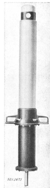
Fig. 3. Kabelendverschluss für 300 kV Prüfspannung.
