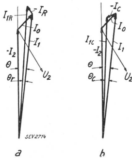
Fig. 8. a Fehrwinkelkorrektur mittels Widerstand. b Fehrwinkelkorrektur mittels Kapazität.
