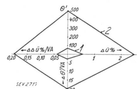
Fig. 11. Allgemeine Charakteristik eines 200/5-A-Wandlers. Bürde = 15 VA, cos phi = 1. 1 Legiertes Eisen. 2 Nickel-Eisen. D = 38 cm, H = 18 cm.
