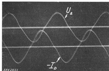
Fig. 41. Oszillogramme für Spannung und Strom der Drosselspule für 5 A. Sekundärstrom.
