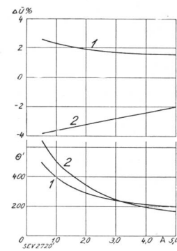
Fig. 14. Fehlerkurven von 200/5-A-Wandlern. D = 38 cm, H = 18 cm. Bürde = 15 VA, \cos \varphi = 1 . 1 Legiertes Eisen. 2 Zweistufenwandler für normale Zähler (Fig. 12c).
