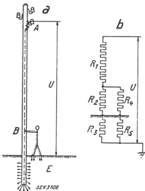
Fig. 6. R_1 Widerstand des Holzmastes zwischen Fehler A und Berührungsstelle B . R_2 Widerstand des Holzmastes zwischen Berührungsstelle B und Erdübergangsstelle. R_3 Erdübergangswiderstand des Holzmastes. R_4 Widerstand des menschlichen Körpers. R_5 Erdübergangswiderstand des menschlichen Körpers.
