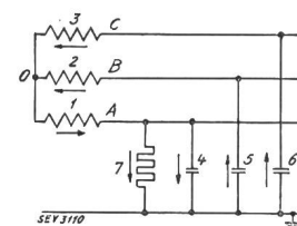
Fig. 8. Widerstandsdiagramm.
