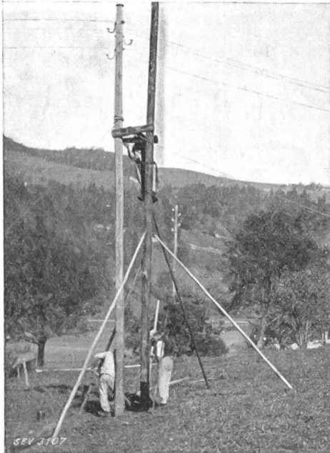
Fig. 5. Der neue Mast wird im Boden verkeilt und mittels Brettern mit dem alten Mast gekuppelt.
