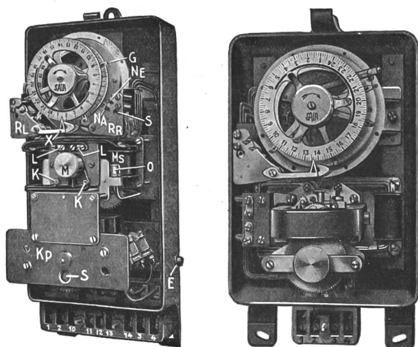
Fig. 8. SAIA-Zeitschalter.
