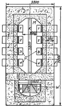
Fig. 19. Cornelius-Versuchsofen in St. Helens (nach Meigh).
