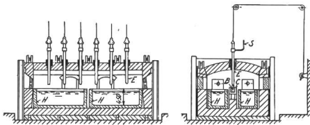
Fig. 5. Lichtbogenofen der A. B. Ugnar nach Maetz.
