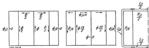
Fig. 3. Verlauf der vertikalen Flusskomponenten.
