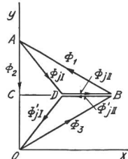
Fig. 2. Flussdiagramm des fünfschenkler Transformators.
