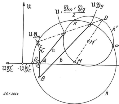
Fig. 3. Graphisch-analytische Berechnungsmethode des Mit- und Gegenstromes: \mathfrak{S}_m = U \cdot \mathfrak{Y}_m \cdot \frac{b}{2a} (Gl. 13) \mathfrak{S}_g = U \cdot \mathfrak{Y}_g \cdot \frac{c}{2a} (Gl. 14) k ist das Kreisdiagramm des zugrundegelegten Zweiphasenmotors, k' ist das Kreisdiagramm der Admittanz \frac{\mathfrak{Y}_m + \mathfrak{Y}_g}{2}
