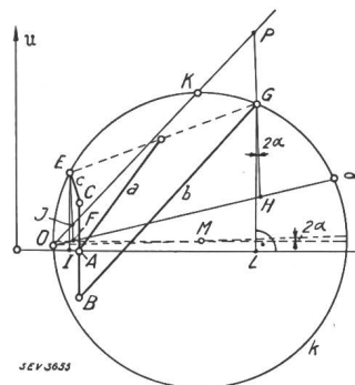
Fig. 4. Bestimmung der Drehmomente und Verluste (s. Gl. 17-22). k ist das Kreisdiagramm des zugrundegelegten Zweiphasenmotors, \overline{O\infty} seine Momentgerade, \overline{OK} seine Leistungsgerade, \text{tg } \alpha = \frac{J_0 R_1}{U} . Der Kreis k' (s. Fig. 3) ist der Uebersichtlichkeit wegen ausgelassen.
