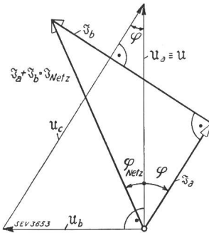
Fig. 2. Vektordiagramm eines C-Motors im «ausgeglichenen» Betriebszustand.
