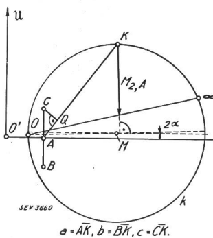
Fig. 10. Anzugs-Drehmoment des C-Motors:
