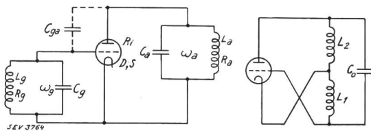
Fig. 5. Huth-Kühn-Schaltung.
