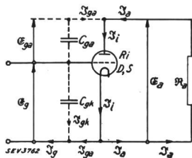
Fig. 1. Schalt-schema.
