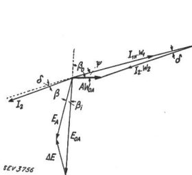
Fig. 2. Stromwandlerdiagramm für Auslösung.
