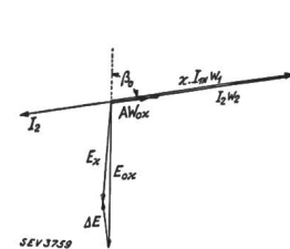
Fig. 6. Stromwandlerdiagramm für Ueberstrom.
