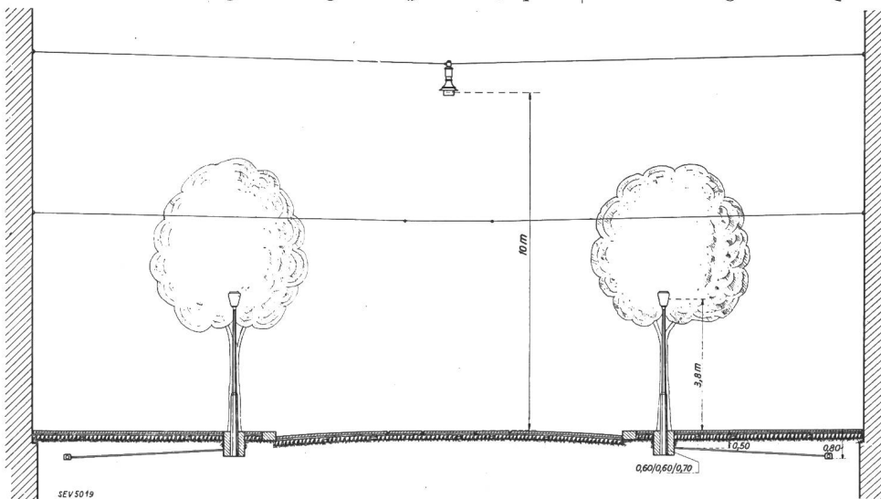
Fig. 25. Querprofil der Bahnhofstrasse.
