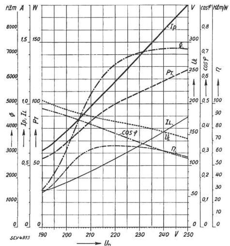
Fig. 3. Betriebscharakteristik der Philora-Natriumdampf-Lampe Typ SO 100 W. Lampe Nr. 4858 mit Streutransformator FKE Nr. 7673. (Kurvenbezeichnung wie Fig. 2.)
