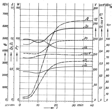
Fig. 2. Anlaufcharakteristik der Philora-Natriumdampf-Lampe Typ SO 100 W bei Nennspannung. Lampe Nr. 4858 mit Streutransformator FKE Nr. 7673. I_p Primärstrom, P_T totale Leistung, U_L Lampenspannung, I_L Lampenstrom, \Phi Lichtstrom, \cos \varphi Leistungsfaktor, \eta Lichtausbeute, f = 50/s .
