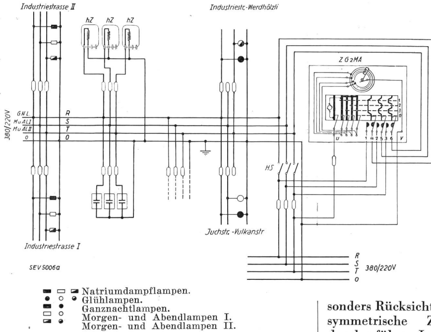
Schalt- und Verteilanlage für die öffentliche Beleuchtung in der Transf.-Station «Industrie».
