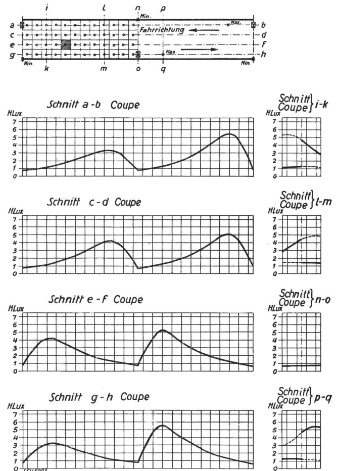
Fig. 10. Vertikal-Beleuchtung an der Industriestrasse. Messebene 1 m über Boden. E_v mittel = 2,5 HLux; E_v max. = 5,4 HLux; E_v min. = 0,7 HLux; Gleichmäßigkeit = 1 : 7,7.
