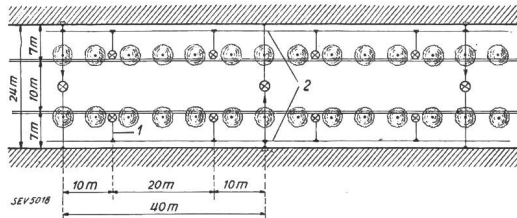
Fig. 24. Situation der Bahnhofstrasse. 1 Kabel 3 \times 1,5 \text{ mm}^2 in 1"-Gasrohr. 2 Kabelleitung 3 \times 25 \text{ mm}^2 in Tonkanal.
