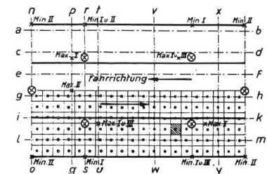
Fig. 27. Vertikal-Beleuchtung der Bahnhofstrasse. Messebene 1 m über Boden. (Kurvenbezeichnung wie Fig. 26.)
