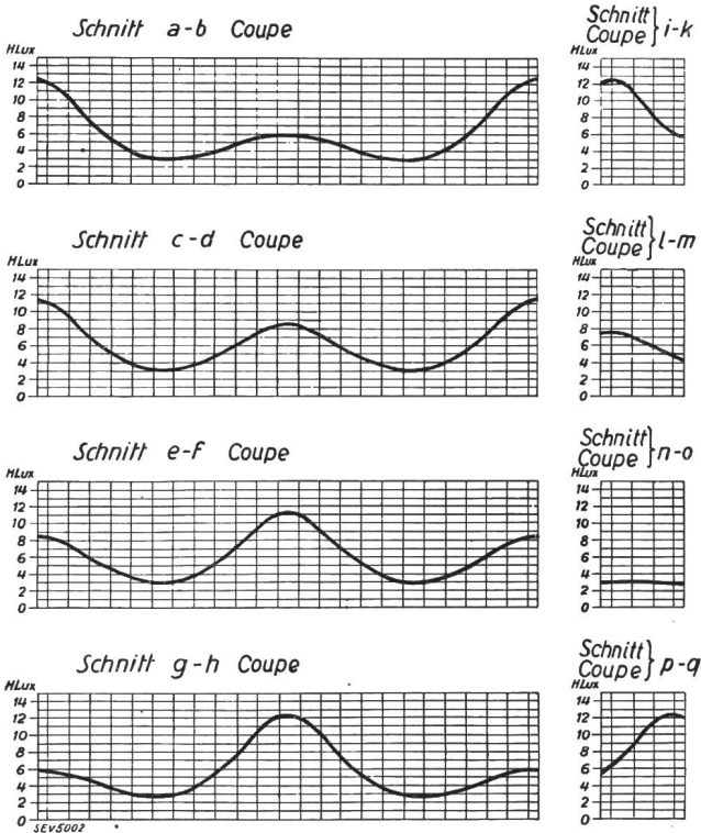
Fig. 9. Horizontal-Beleuchtung an der Industriestrasse. Messebene 1 m über Boden. E_h mittel = 5,9 HLux; E_h max. = 12,4 HLux; E_h min. = 2,8 HLux; Gleichmäßigkeit = 1 : 4,4.
