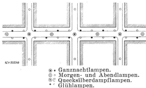
Fig. 30. Schaltbild der Bahnhofstrasse.
