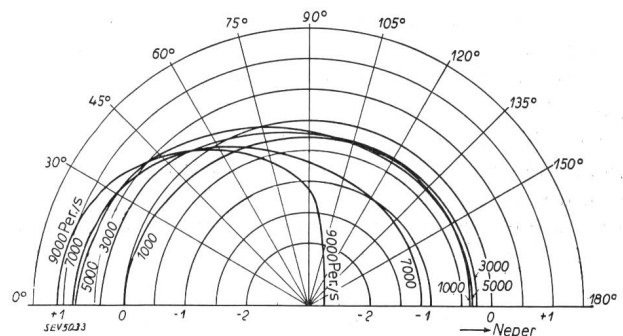
Fig. 4. Kondensator-Mikrophon. Telefunken ELA M 14 (Kapsel CM 5 Nr. 55).
