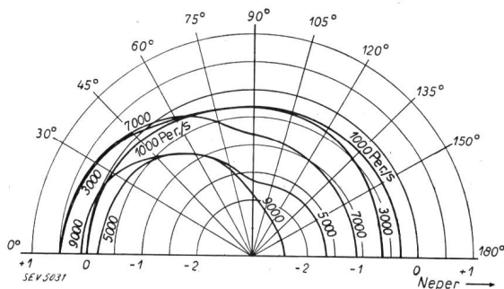
Fig. 2. Moving Coil-Mikrophon. Standard Telephone & Cables, 4017 A (Nr. 328).
