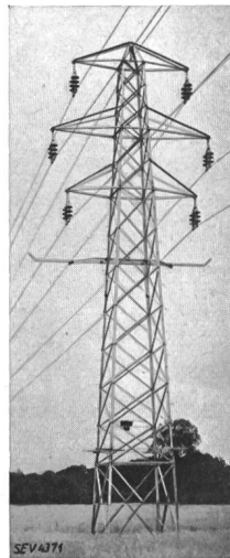
Fig. 5 a. Strassenüberkreuzungsmast mit Doppelaufhängung und «Erdungstraverse». (Photo Henley.)
