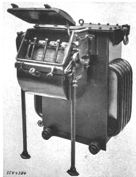
Fig. 17. Transformator, mit Schalter und Sicherungen zusammengesetzt. Der Schalterdeckel kann nur bei ausgeschaltetem Schalter geöffnet werden; die Sicherungen können von Hand ersetzt werden, da das Schalterinnere durch Isolierplatte abgedeckt ist. (Brush, Ltd. Longborough.)
