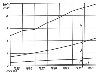
Fig. 6. Energieabgabe in den Jahren 1925 bis 1931. 1 für öffentliche Be- leuchtung. 2 für Bahnbetrieb. 3 für Beleuchtung u. Haushalt. 4 für Motoren.
