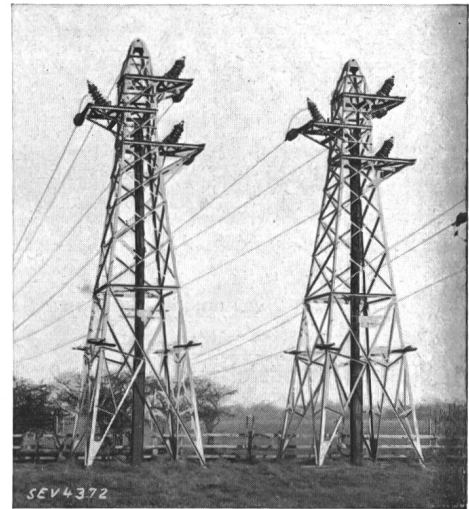
Fig. 5 b. 33 kV «Grid»-Sekundärleitungen. Kabel-Endmasten. (Photo CEB.)
