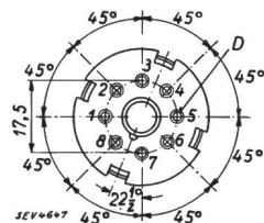
Abmessungen der Typen 6A8, 6J7, 6K7. A Gitteranschluss. B Metall-Abschirmung. C Metall-Grundplatte. D Kontaktstift.
