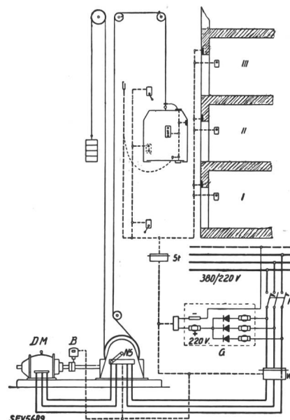
Fig. 1. Schematische Darstellung eines mit Gleichrichter für die Steuerung umgestellten Aufzuges. — Arbeitsstromkreis (Drehstrom), --- Steuerstromkreis (Gleichstrom), HS Ueberstrom-Hauptschalter, WS Wendeschalter, NS Wendeschalter, DM Drehstrommotor, G Trockengleichrichter, B Bremslüftmagnet, ST Stockwerkschalter.
