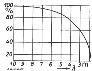
Fig. 3. Abnahme der Durchsteuerung mit der Wellenlänge.
