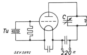
Fig. 2. Schema des Senders.
