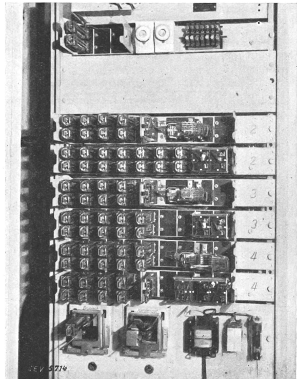
Fig. 15. Empfangsapparatur der Fernmeldeanlage.
