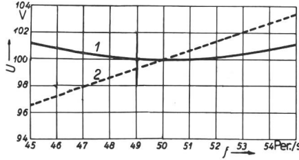
Fig. 3. Frequenzabhängigkeit.
