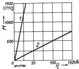
Fig. 2. Energieverbrauch. 1 Neues System, mit Rotor aus Eisen-Kupfer-Kombination, ohne inneren (feststehenden) Eisenkern. 2 Uebliches System mit Aluminiumtrommel und feststehendem Rotorkern.
