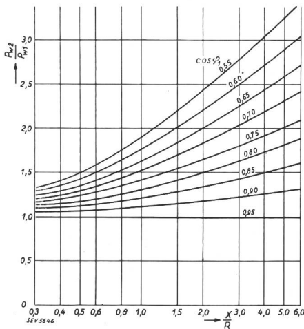
Fig. 4. Verhältnis der Wirkleistungen bei Phasen-schiebung von \cos \varphi (nacheil.), auf \cos \varphi_2 = 0,95 .
