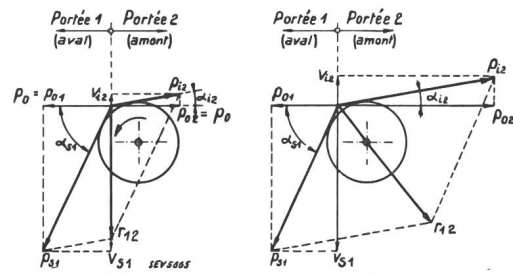
Fig. 3. Equilibre stable d'une poulie libre: p_{s1} = p_{i2}
