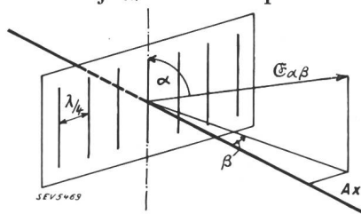
Fig. 4. Strahlwerfer mit q parallelen Dipolen, in einem Abstand von je \lambda/4 .
