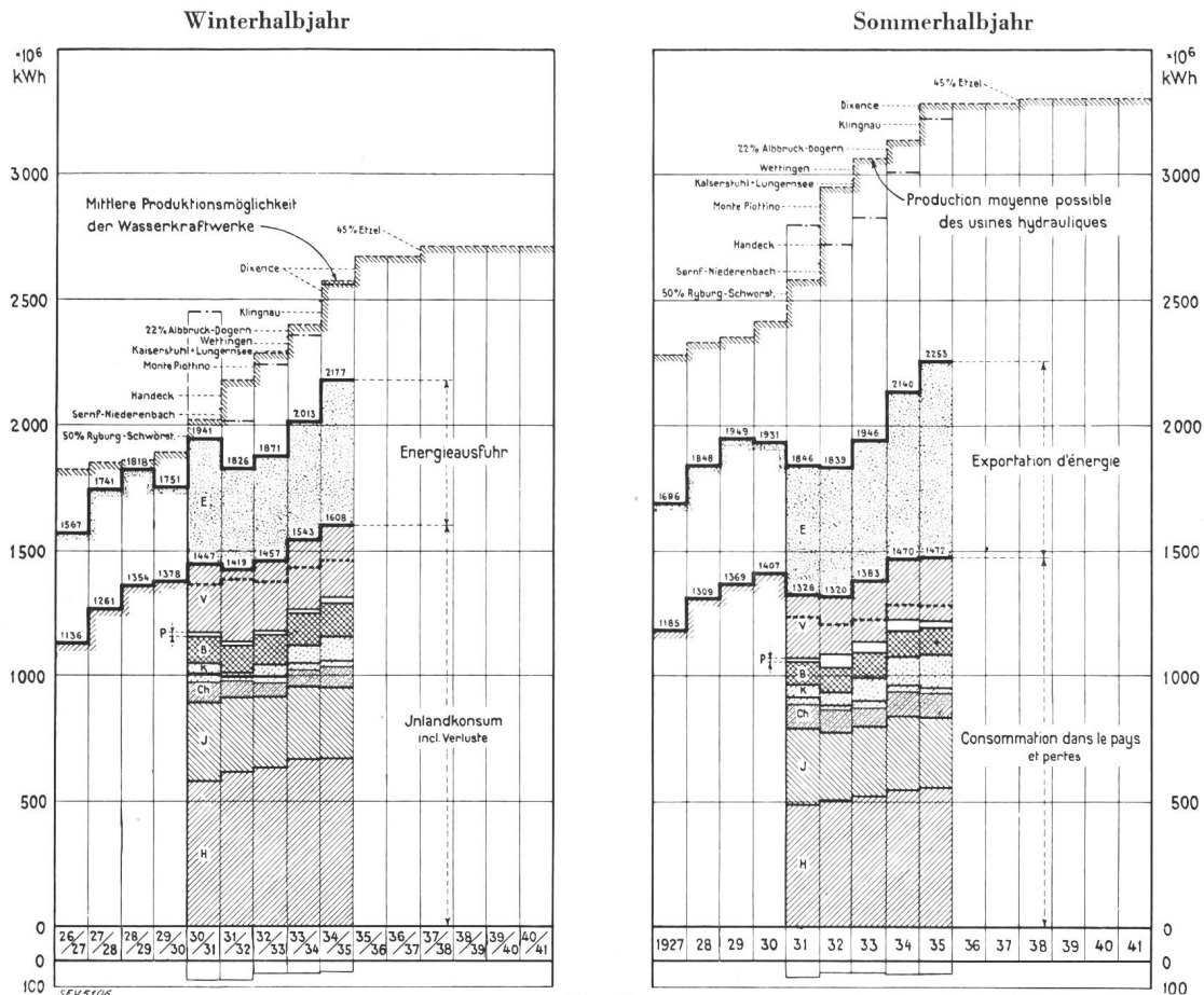
Fig. 2. Mittlere Produktionsmöglichkeit, Inlandkonsum und Energieausfuhr. H Haushalt und Gewerbe. J Allgemeine Industrie. Ch Elektrochemische, -metallurgische u. -thermische Anwendungen. K Elektrokessel. B Bahnen. P Pumpenspeicherung. V Verluste. E Energieausfuhr.
