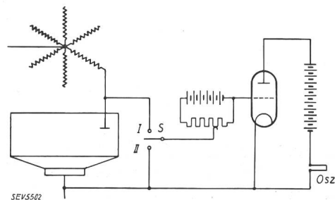
Fig. 1. Os2 Oszillograph.
