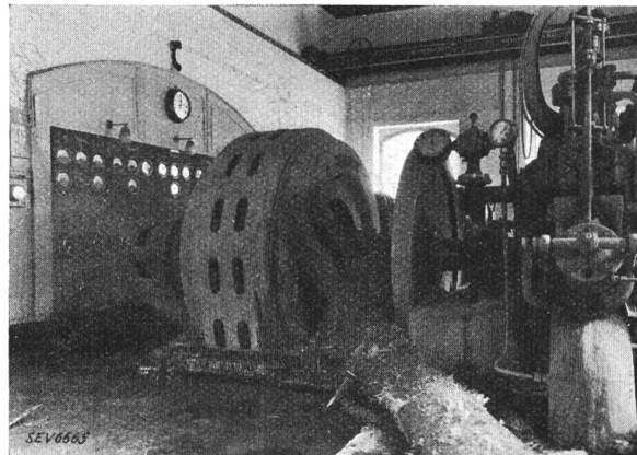
Fig. 11. Baumstämme in Generatoren.
