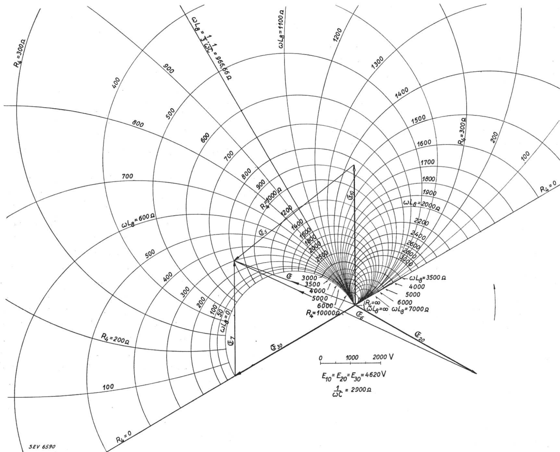
Fig. 10. Direkter Erdschluss über ohmschen und induktiven Widerstand. Ortskurven der Polleiter-EMKe gegen Erde.
