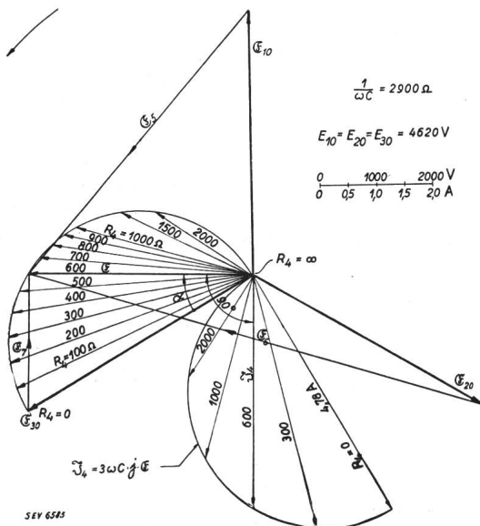
Fig. 5. Direkter Erdschluss über ohmschen Widerstand. Ortskurve der Spitzen von \mathcal{E} und \mathcal{J} .
