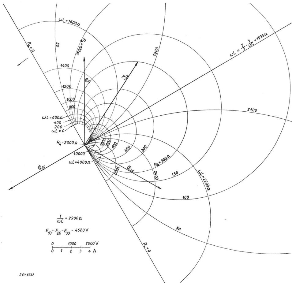
Fig. 15. Indirekter Erdschluss. Ortskurven des Erdschlußstromes.
