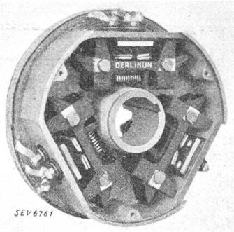
Fig. 8. Oerlikon Zentrifugalanlasser 1927 mit Scherenschalt elementen.
