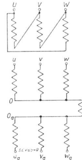
Fig. 2. Sechshephasenschaltung mit Saugdrosselspule.
