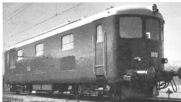
Fig. 3. Dieselelektrische Lokomotive Am 4/4 1001 der SBB. Dauerzugkraft am Radumfang 3090 kg bei 72,5 km/h. Höchstgeschwindigkeit 110 km/h.
