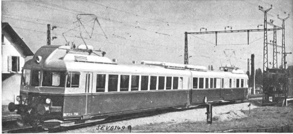
Fig. 1. Leichttriebzug Typ BCFZe 4/6 der BLS. Zugkraft einstündig 3320 kg bei 68,5 km/h. Höchstgeschwindigkeit 110 km/h.
